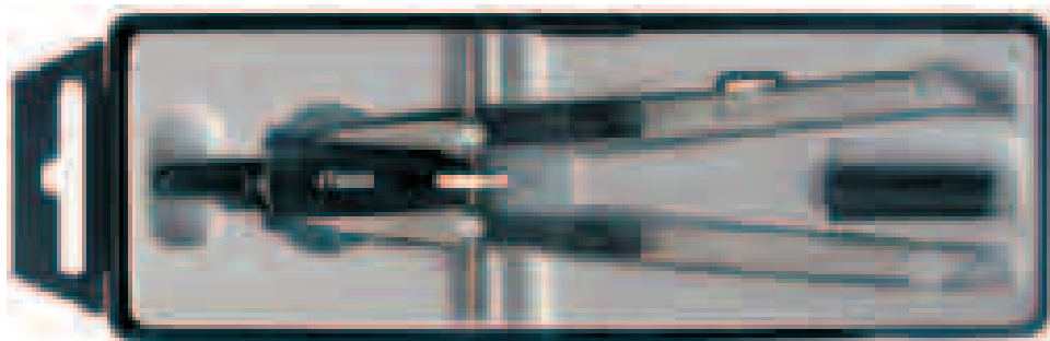
Schnellverstellzirkel 170 mm, Hebelmechanik, Kreise bis 370 mm, 2 knickbare Gelenke, geeignet für Zirkeleinsatz 4 mm, Minendose, Klarsichttui
